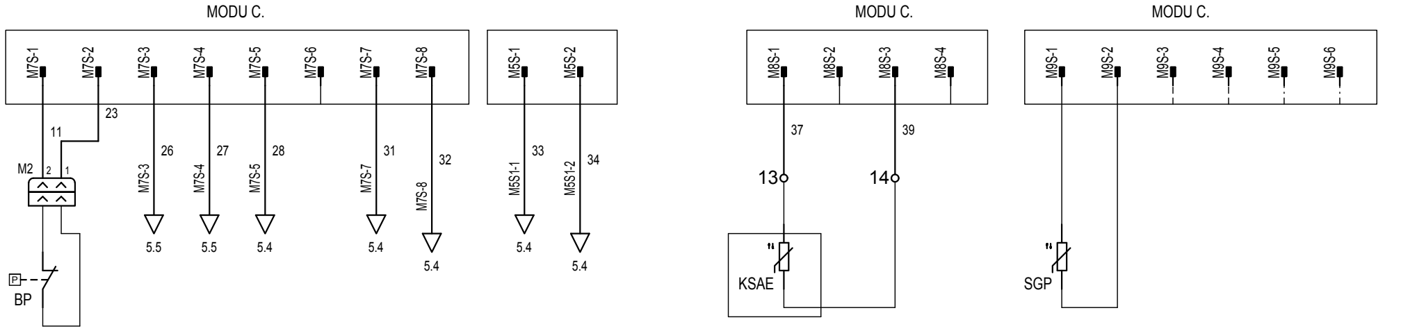
SONDA AMBIENTE ESTERNO AMBIENT AIR TEMPERATURE PROBE
