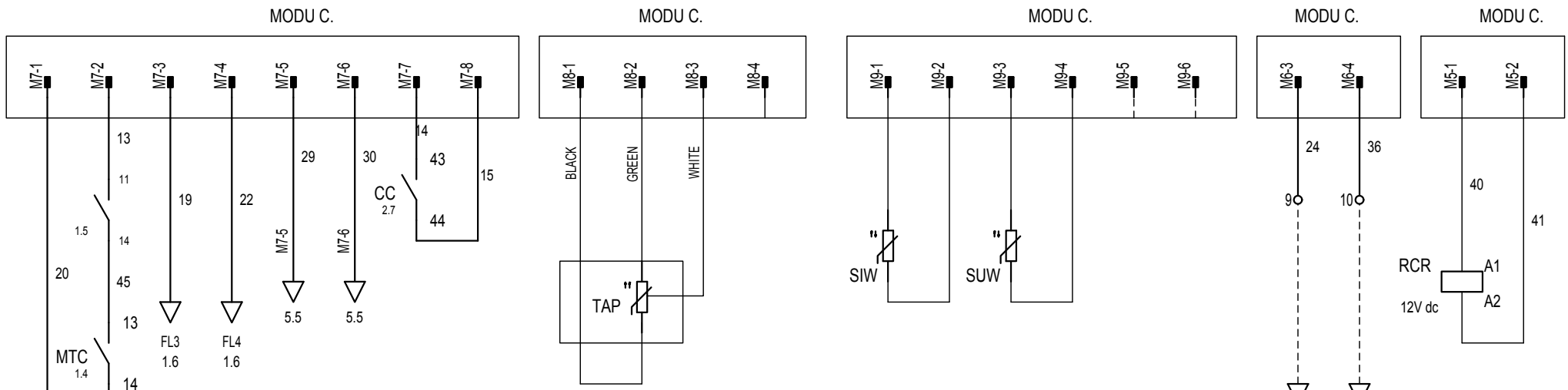
SONDA AMBIENTE ESTERNO AMBIENT AIR TEMPERATURE PROBE
