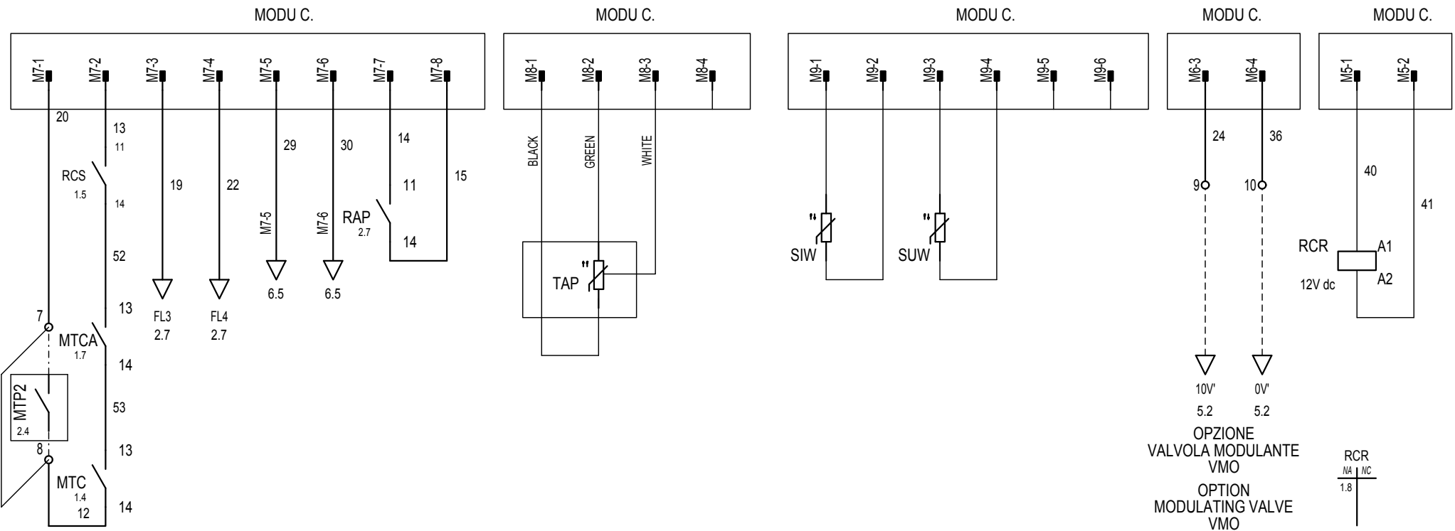
SONDA AMBIENTE ESTERNO AMBIENT AIR TEMPERATURE PROBE
